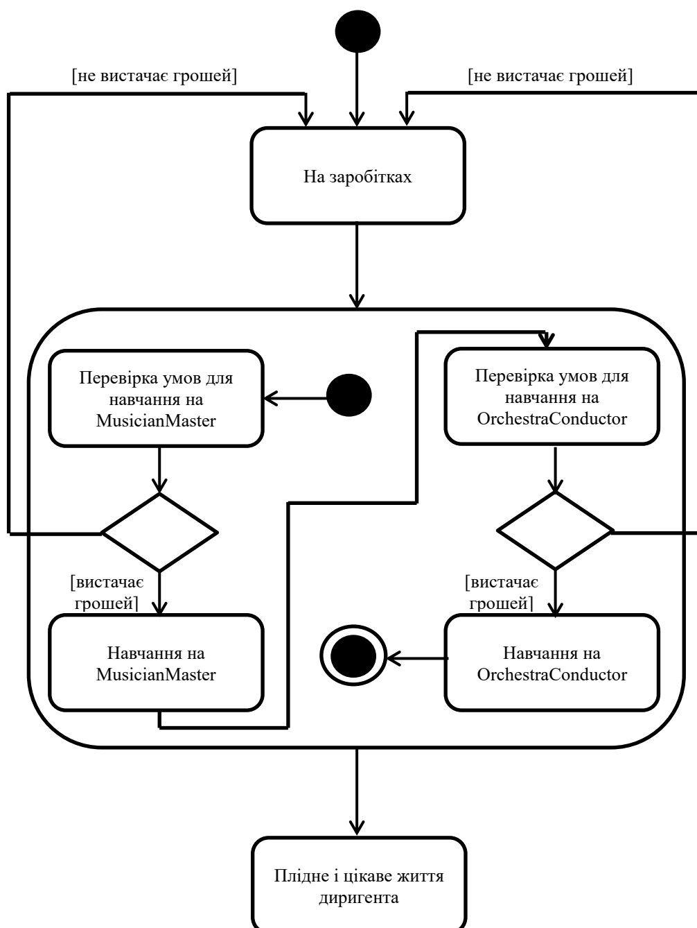
Рисунок 3.7 – Діаграма станів
