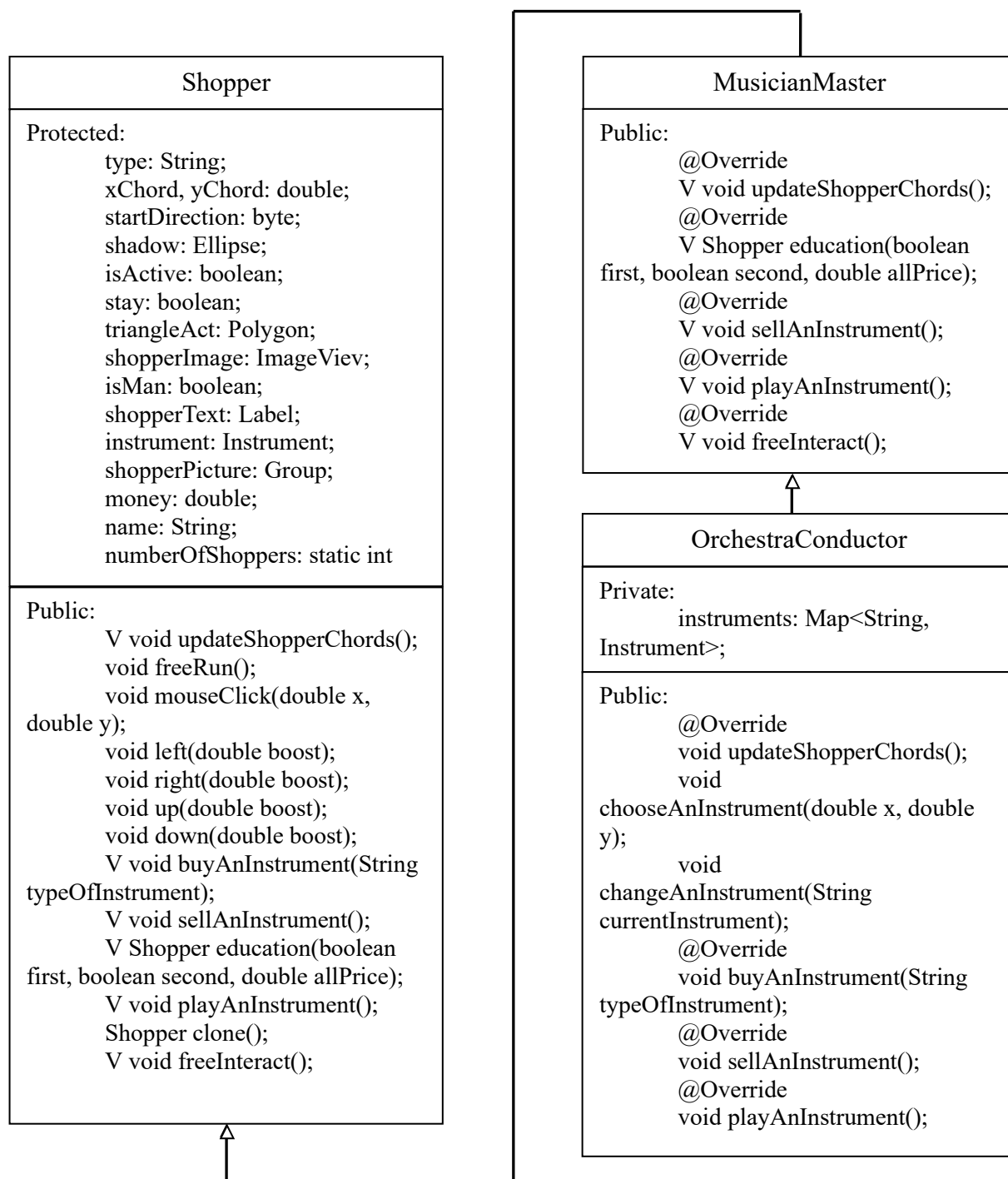
Рисунок 3.1 – Діаграма наслідування
